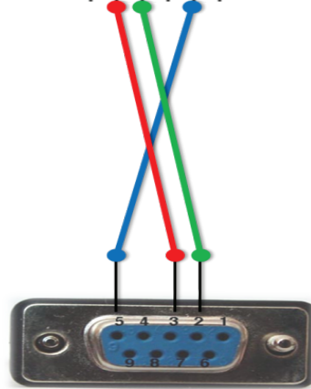
DB9 Hembra – Vista frontal del conector
