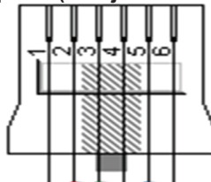
RJ25/RJ11 – Vista superior de los pines (clavija hacia abajo)
