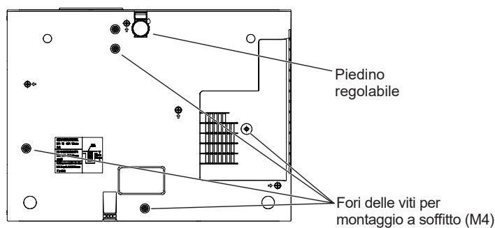
Posizione dei fori delle viti per il montaggio a soffitto e del piedino regolabile
